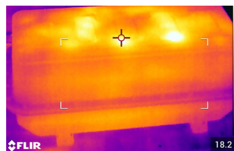
Figure 9. Un bloc-batterie durant un cycle de charge
