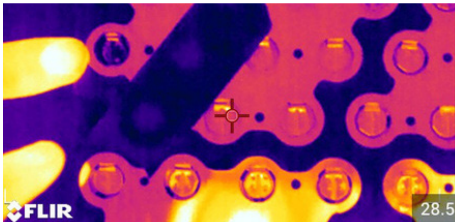
Figure 7. Identification des fuites cellulaires à l'aide d'une caméra FLIR de la série T
