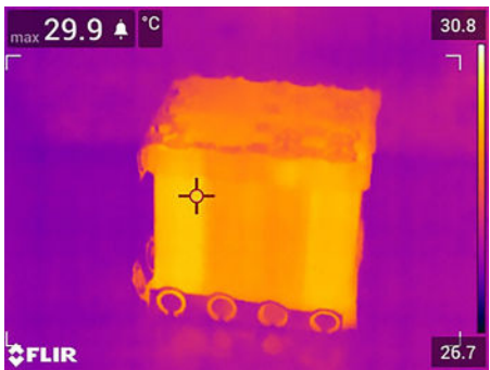
Figure 2. Image thermique d'un bloc-batterie composé de cellules LI-ion
