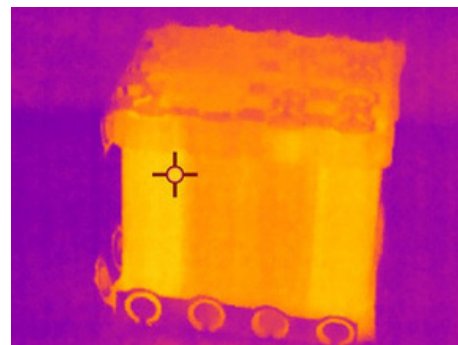
Figure 8. Température irrégulière affichée par la batterie au lithium
